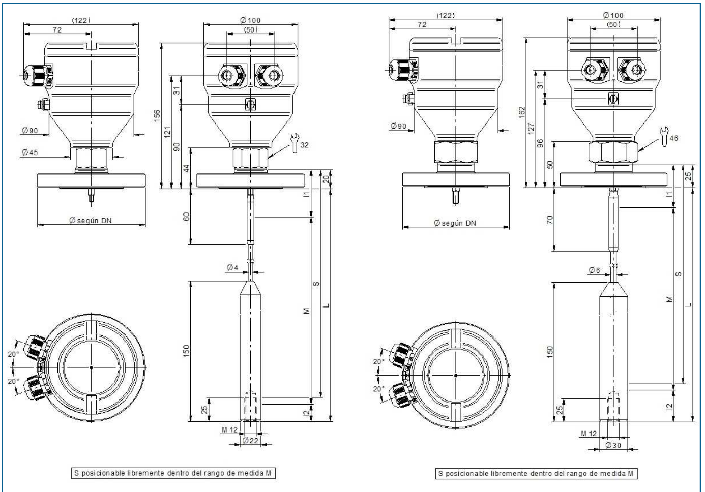
Fig. 9. Sonda cable — conexión brida
