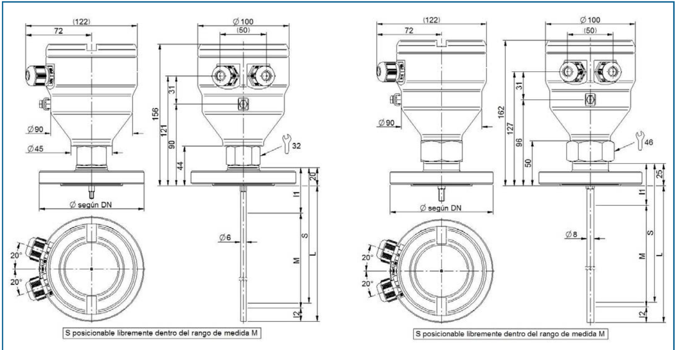
Fig. 7. Varilla simple — conexión brida
