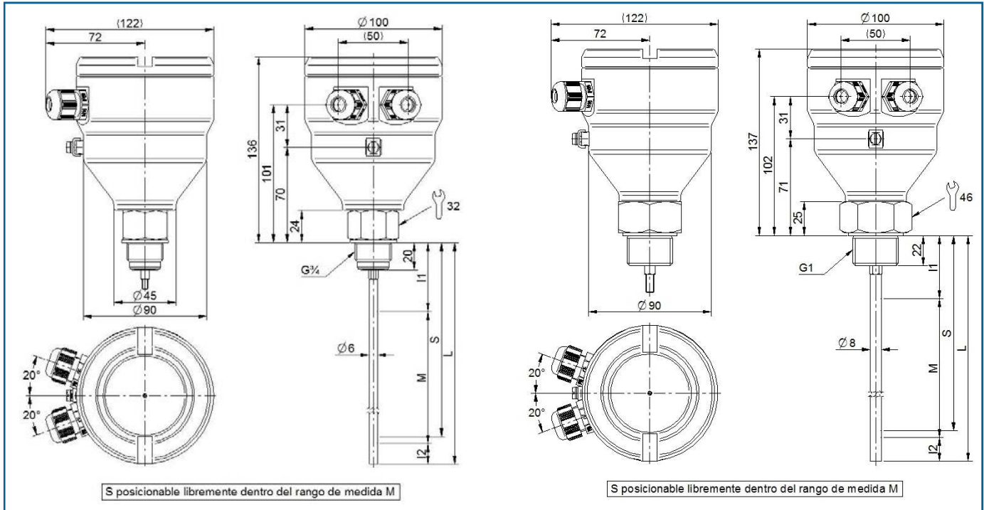
Fig. 3. Varilla simple
