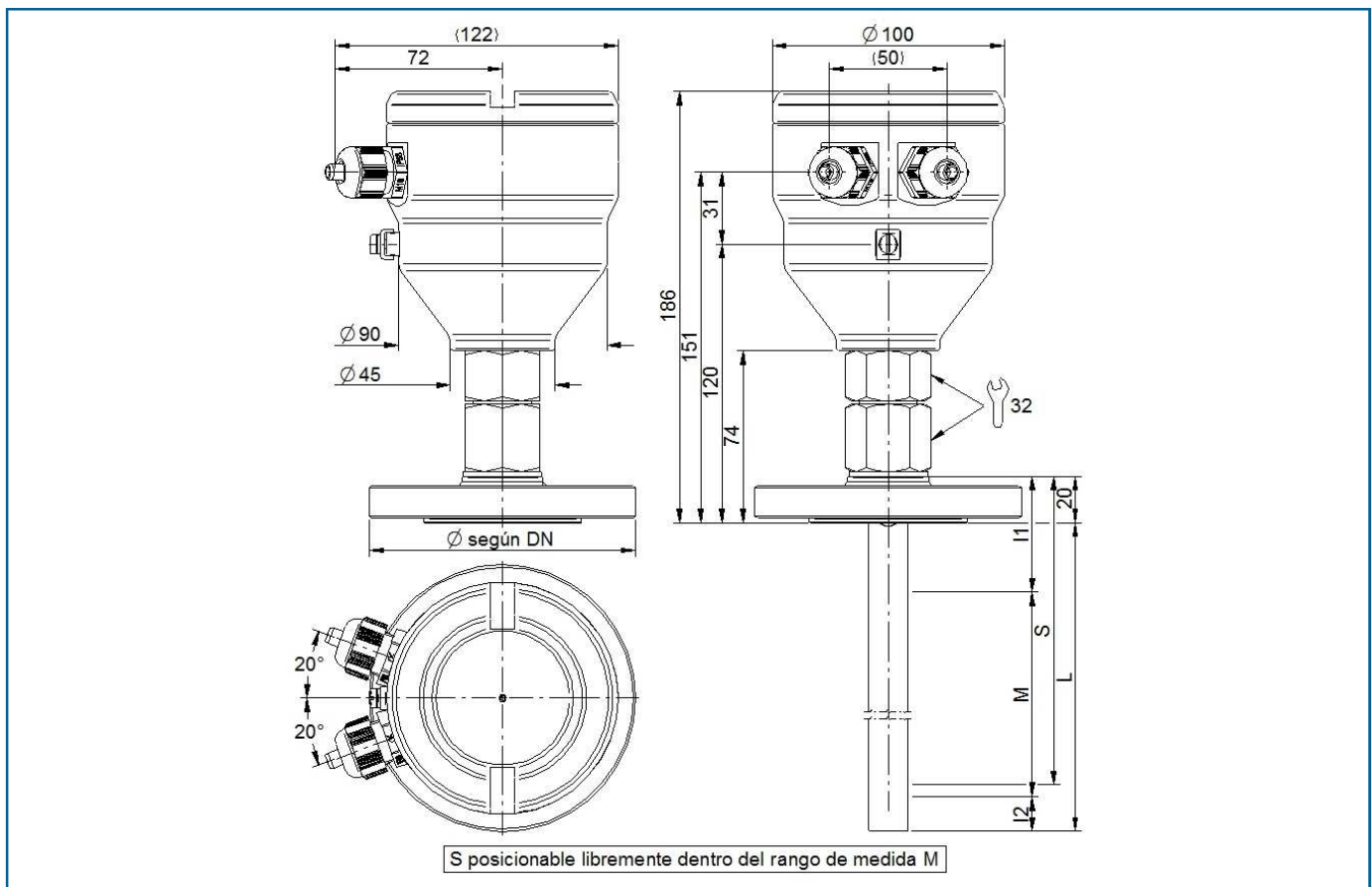
Fig. 8. Sonda coaxial — conexión brida
